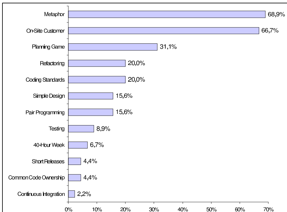
Abbildungung 51: Am wenigsten benutzte Elemente (n=45)
