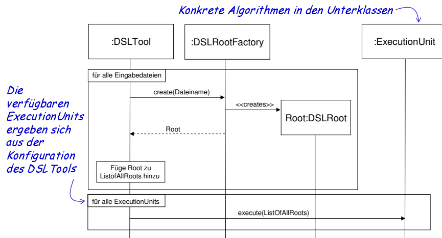
Abbildung 3.4.: Ablauf der Verarbeitung innerhalb eines DSLTools
