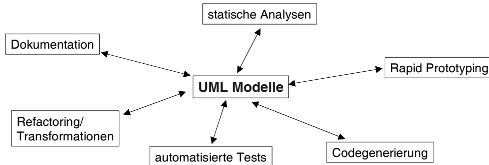
Abbildung 1.1.: Modellbasierte Softwareentwicklung
